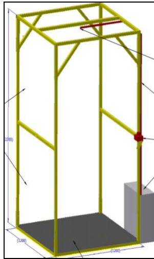
Gambar 1. Rancangan Bilik Sterilisasi ( Smart Sterilization Booth )
