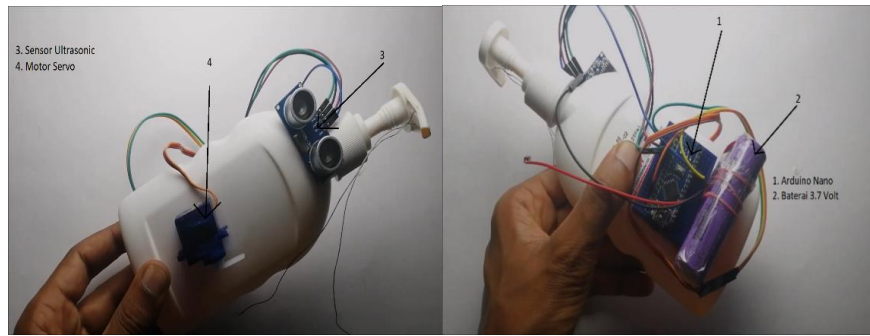
Gambar 6. Rancangan Rangkaian Sensor Tempat Sabun
